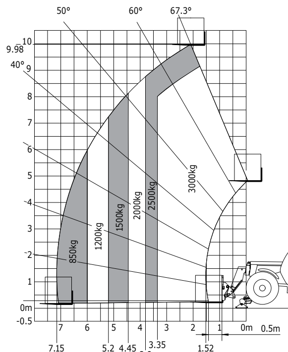
Maschine mit Gabeln auf Stützen CDG 500 mm
